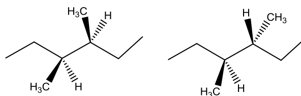
diastereomeren
