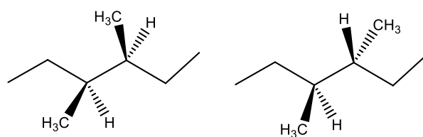
diastereomeren
